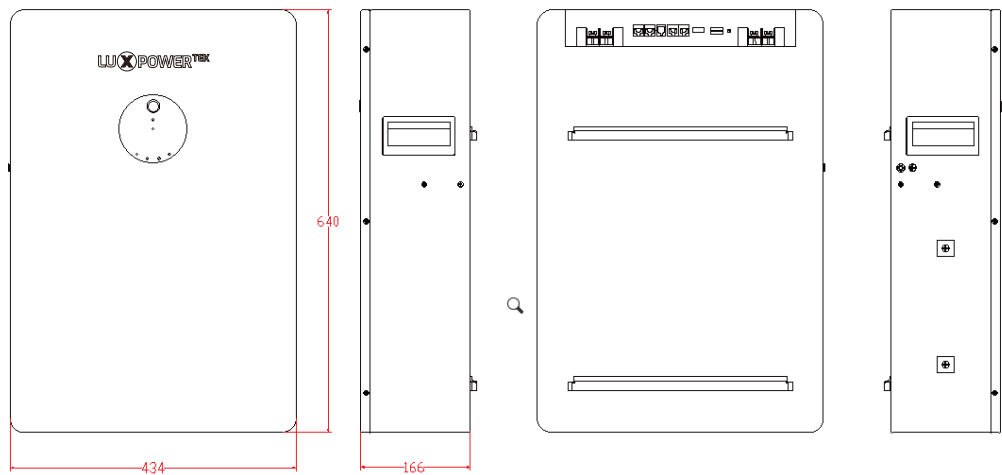
Figura 3-2 Dimensões do produto:
